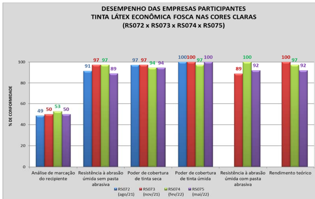
Figura 5 - Evolução das empresas PARTICIPANTES para cada análise de tinta látex econômica realizada no âmbito do Programa de Qualidade
